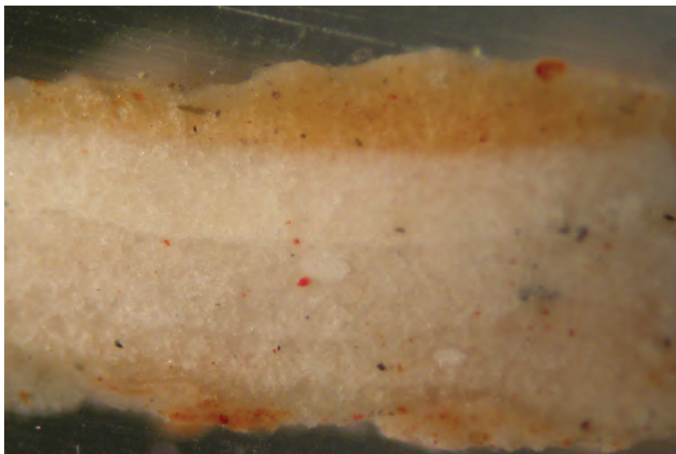
47. ŠMARTNO NA POHORJU (ŠP VII) – prečni prerez vzorca inkarnata sv. Nikolaja: oranžna podslíkava, več belih nanosov, oranžna plast linije senčenega nosu (x200)
