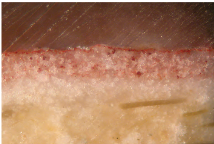
7. BRDINJE (BRD 2) – prečni prerez vzorca draperije: omet, belež, osnovna svetlordeča plast, čez tanka rdeča modelacija (x200)
