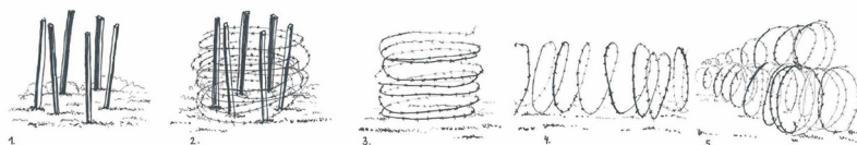
Slika 4: Stanislav Sluga iz Dolenje Brezovice je sodeloval pri postavljanju zapore meje z NDH pod Gorjanci. Skica prikazuje način postavljanja pasu bodeče žice, kot se ga spominja.
