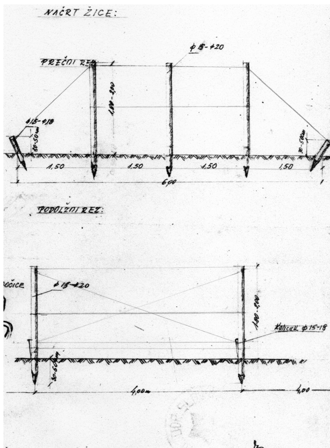
Slika 3: Prečni in podolžni načrt pasu bodeče žice, ki ga je narisal obveščevalec Vzhodnodolenjskega odreda, 10. julij 1943.
