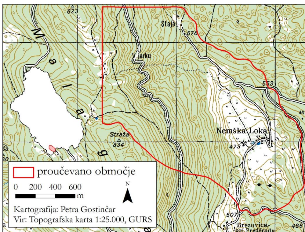
Slika 29: Pregledna karta Nemške Loke
